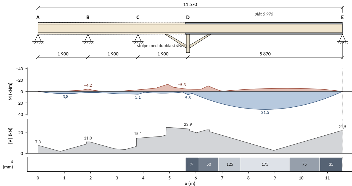
Figur 2: Nockbalk 1. Stöd, plåtbitar, omhüllande moment (ritat på dragen sida) och tvärkraft i brottgränstillstånd för samtliga modeller och lastfall, med och utan limverkan, samt skruvdelning s längs plåten (mm).
