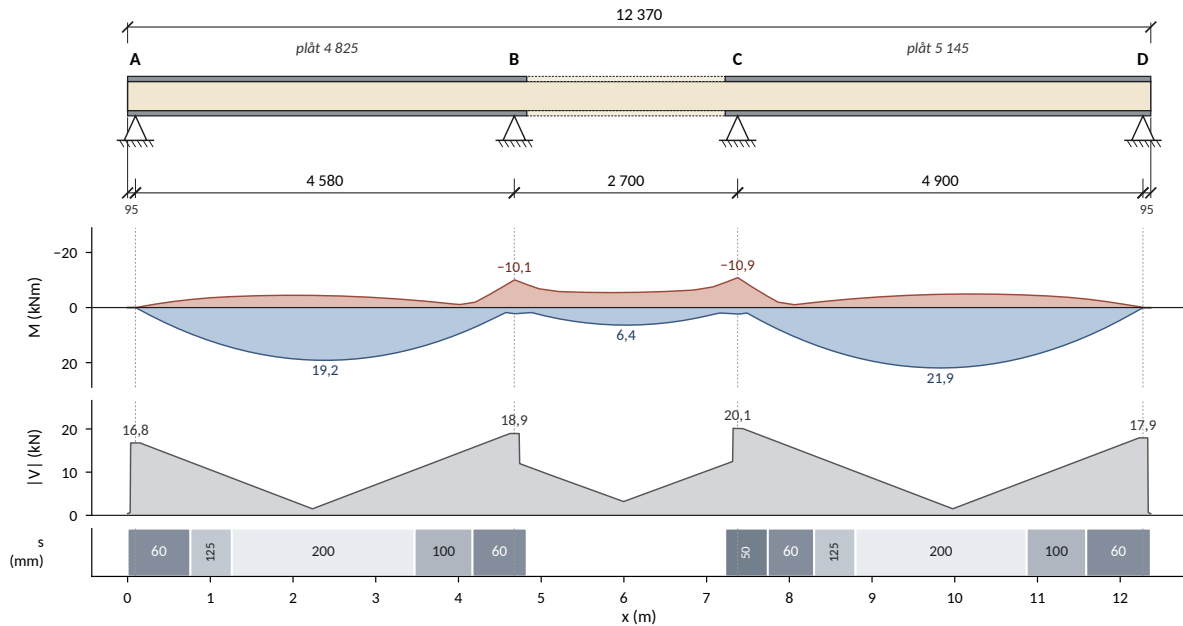
Figur 6: Nockbalk 5. Stöd, plåtbitar, omhullande moment (ritat på dragen sida) och tvärkraft i brottgränstillstånd för samtliga modeller och lastfall, med och utan limverkan, samt skruvdelning s längs plåten (mm).
