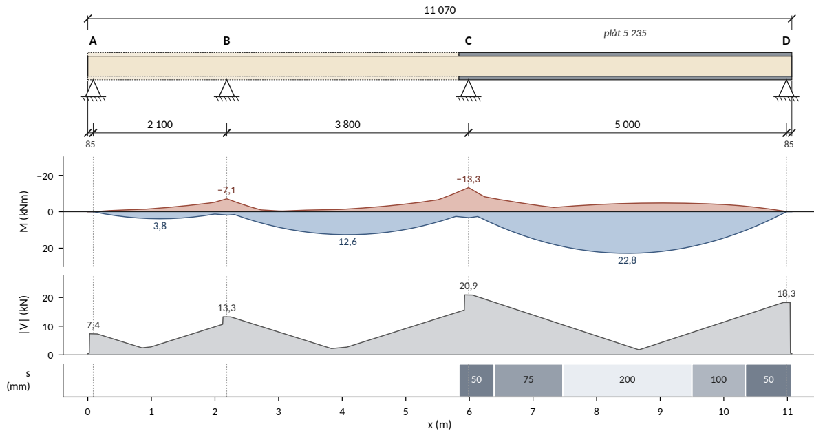
Figur 4: Nockbalk 3. Stöd, plåtbitar, omhüllande moment (ritat på dragen sida) och tvärkraft i brottgränstillstånd för samtliga modeller och lastfall, med och utan limverkan, samt skruvdelning s längs plåten (mm).
